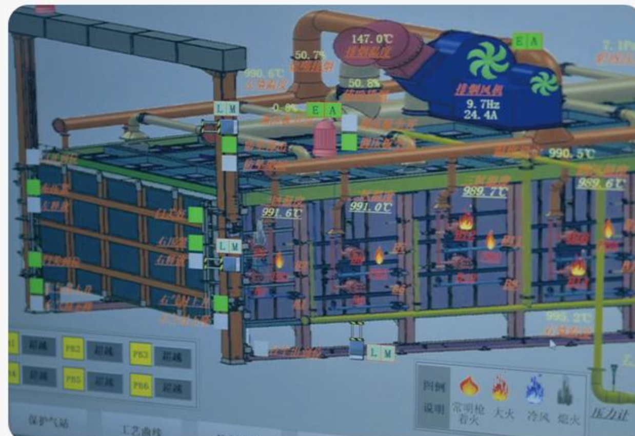
行业首创台车炉 再结晶退火工艺
